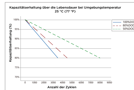
5 kWh LFP-Batterie
