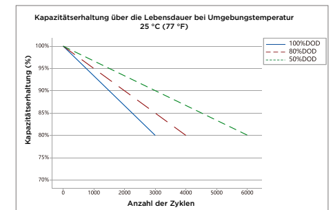
2 kWh LFP-Batterie
